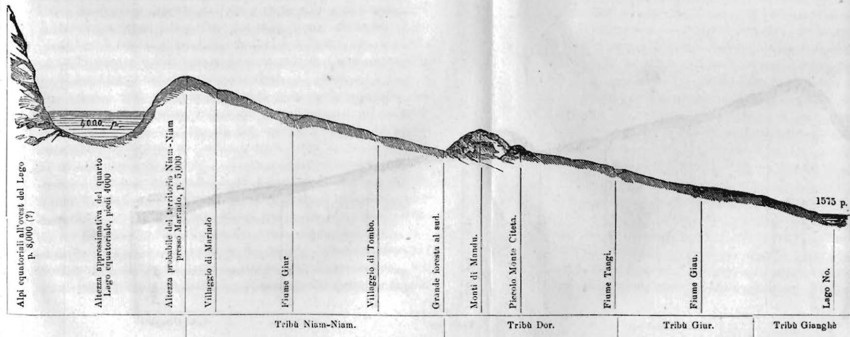
Profilo longitudinale secondo la linea A B.
