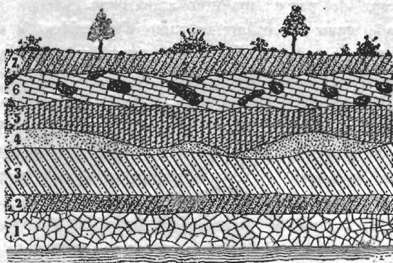
FIG. 2ª — Stratificazione sul Lago Buscioftù.
