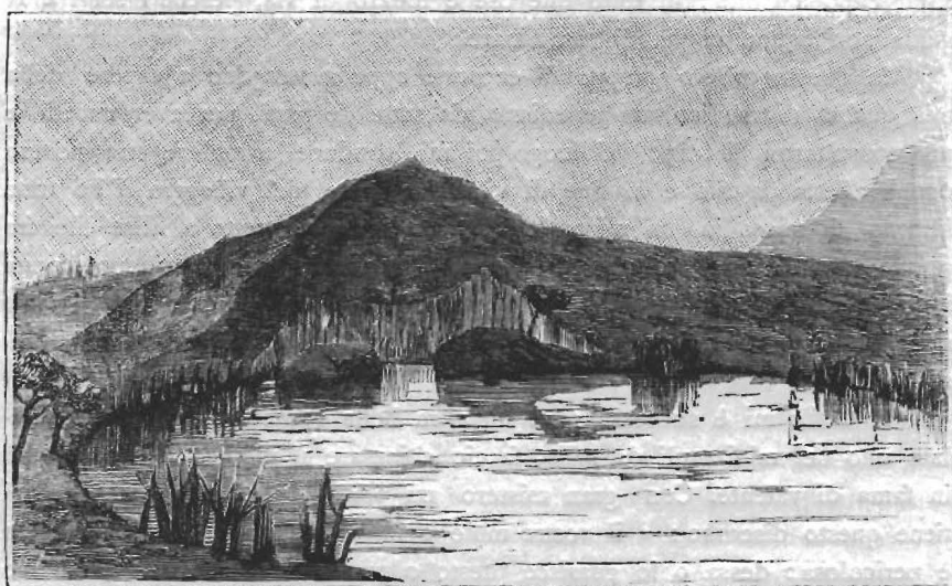
FIG. 1 a — Lago Kilolé.
