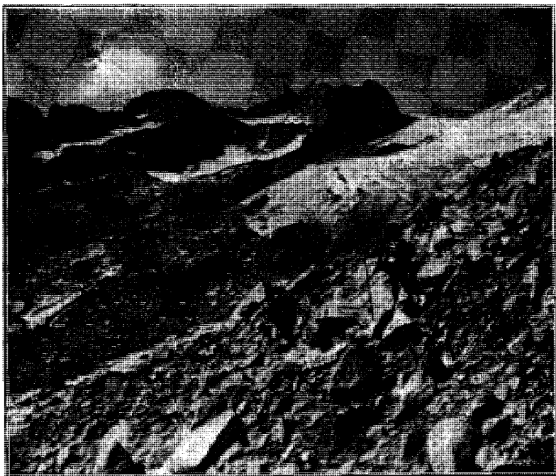
FIG. 3ª — Lingua del ghiacciaio del Nardis. (Anno 1911).
