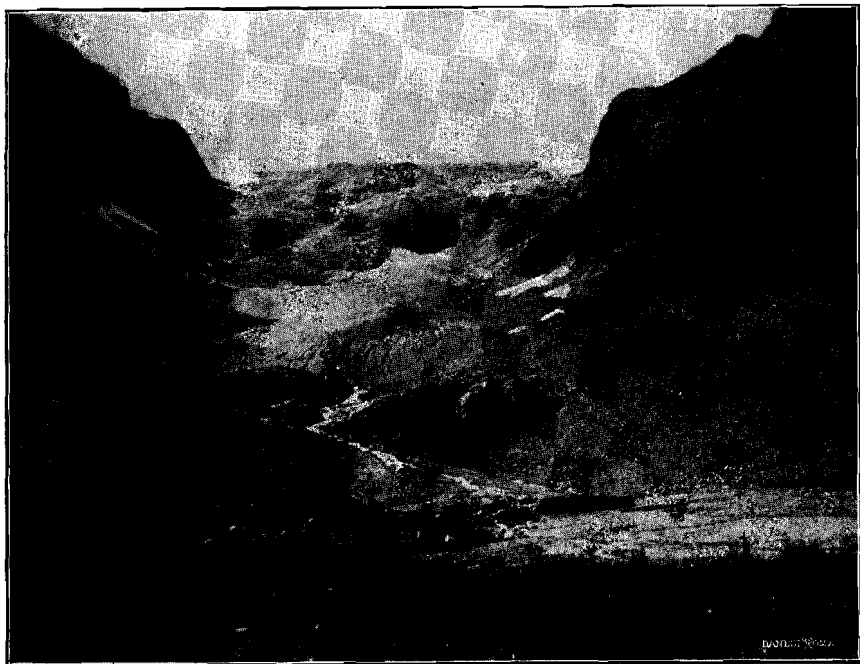
FIG. 2 a — Lingua del ghiacciaio del Lobbia. (Anno 1911).
