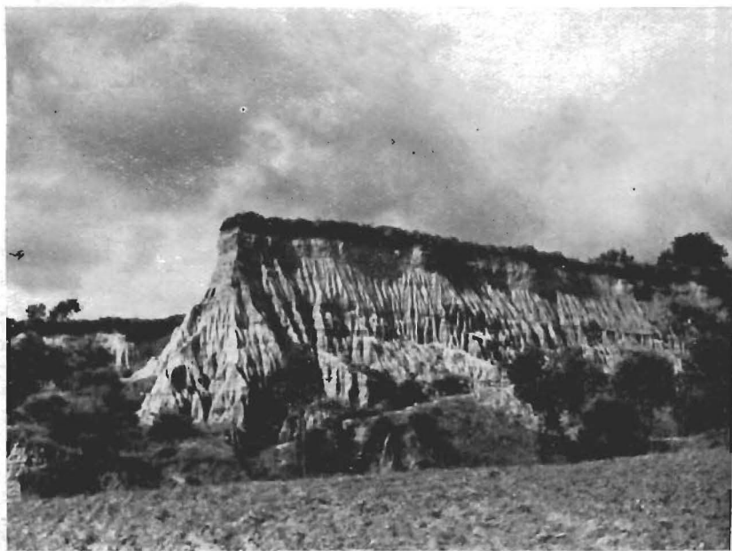
Forme d'erosione nelle argille tra Diamante e Belvedere Marina. (Cosenza).
