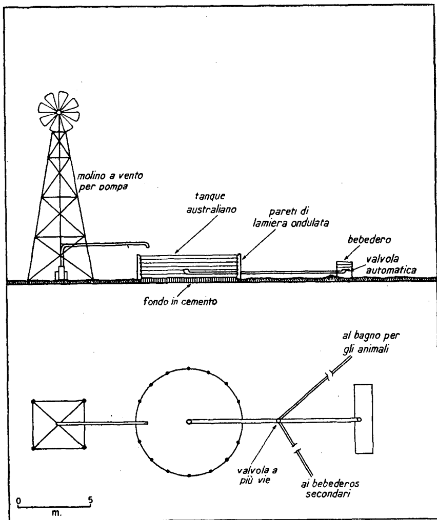
FIG. 3. — LE INSTALLAZIONI DI UN « TANQUE AUSTRALIANO » VISTE IN SEZIONE E IN PIANTA.
