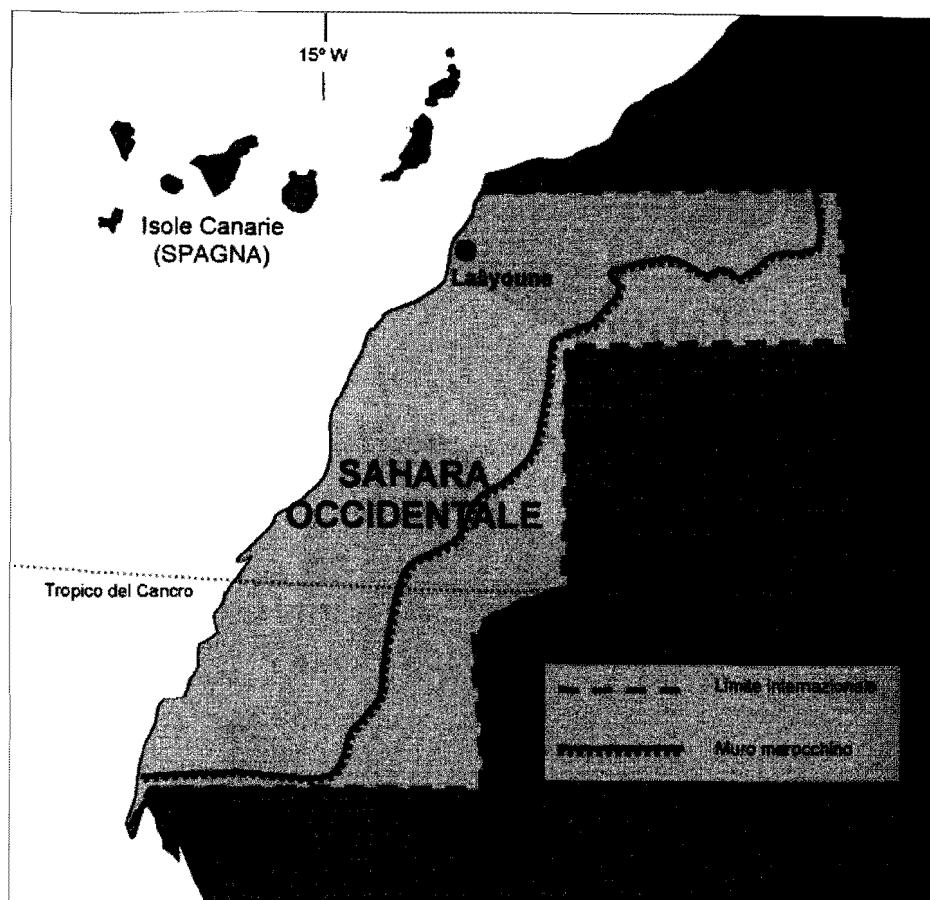
Fig. 1 – Occupazione territoriale marocchina nel Sahara Occidentale
