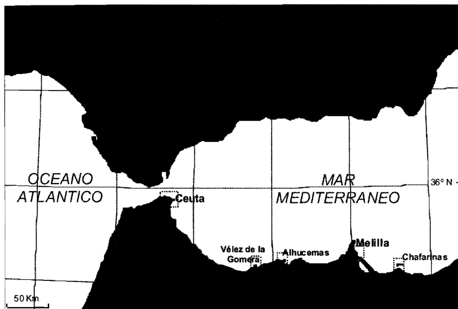
Fig. 3 – Possedimenti spagnoli lungo la costa dell'Africa settentrionale
