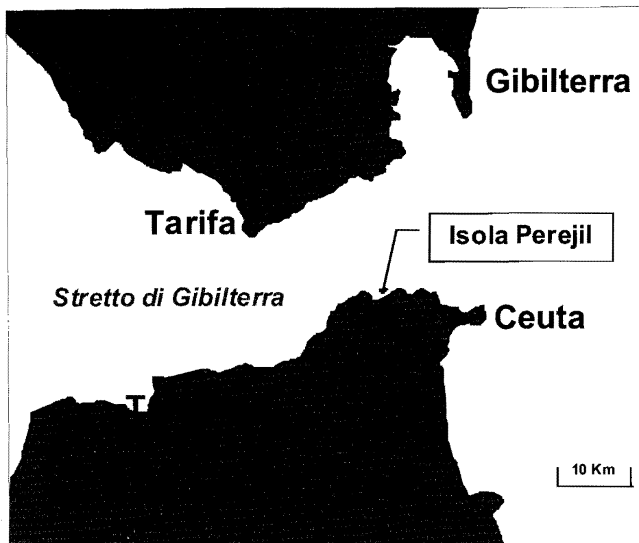
Fig. 2 – Ubicazione dell'isolotto di Perejil nello Stretto di Gibilterra
